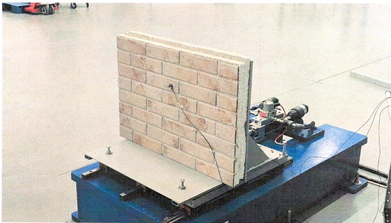
Рисунок 1 Общий вид изделия, закрепленного на платформе вибростенда. При воздействии горизонтально, перпендикулярно лицевой стороне (ось OX).
