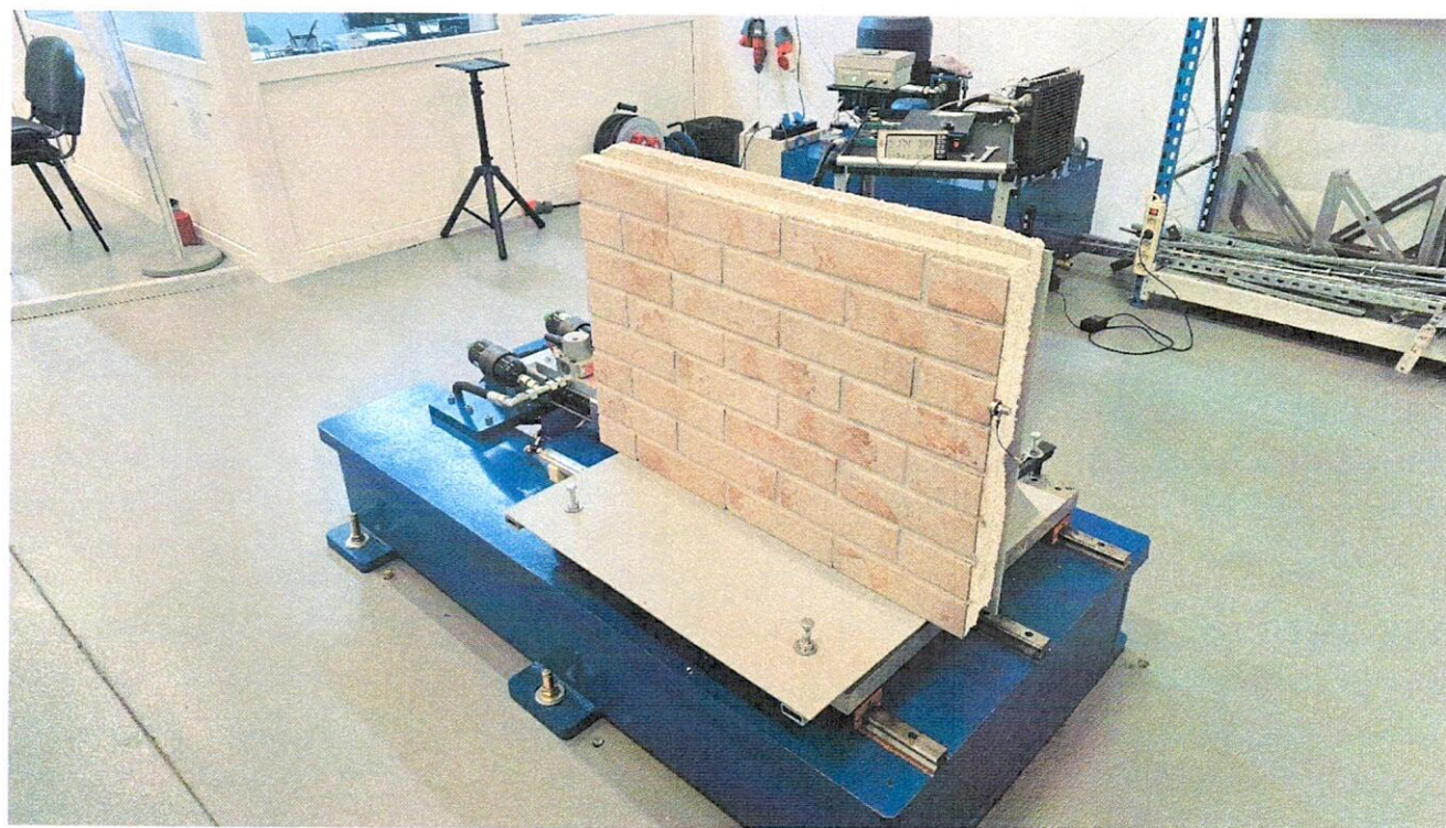
Рисунок 2 Общий вид изделия, закрепленного на платформе вибростенда. При воздействии горизонтально, параллельно лицевой стороне изделия (ось OY).
