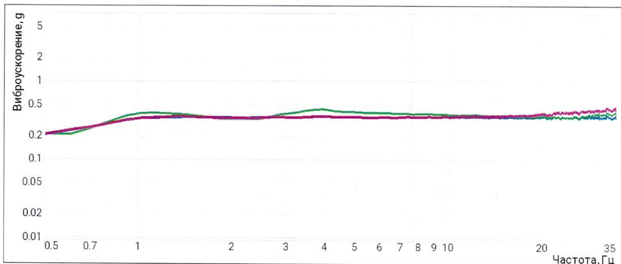
Рисунок А1 – Испытание на сейсмостойкость уровня ПЗ. Направление воздействия, горизонтальное по оси ОХ.
