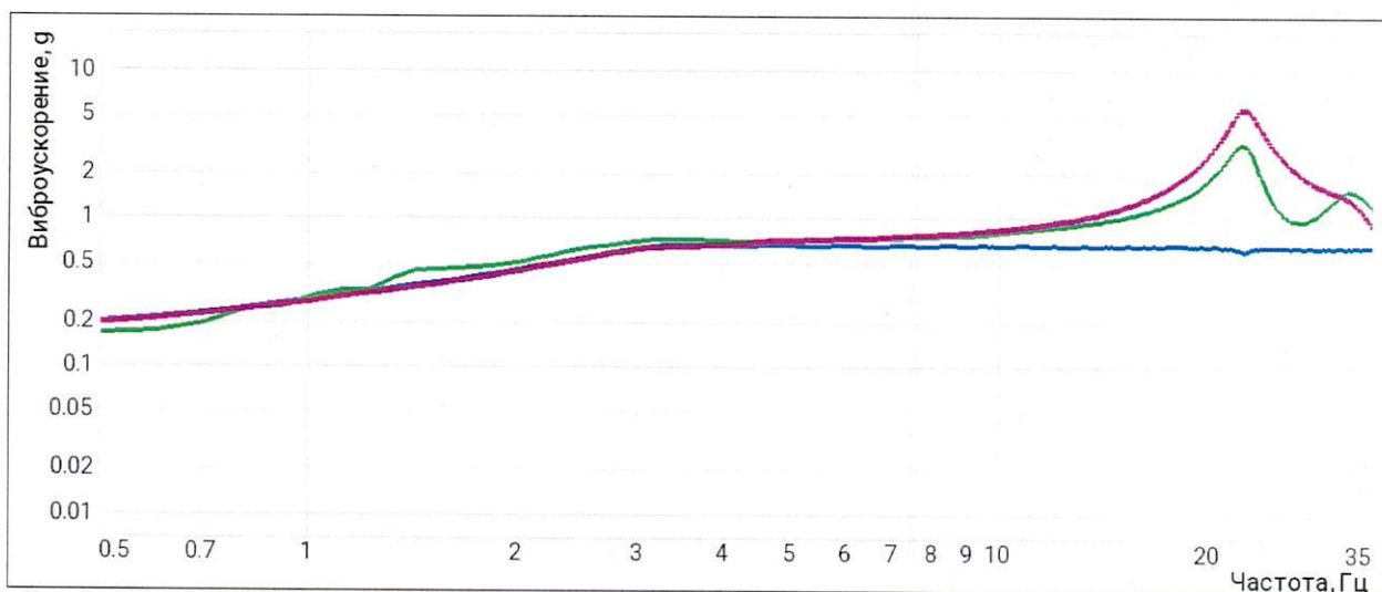
Рисунок А3 – Испытание на сейсмостойкость уровня ПЗ. Направление воздействия, вертикальное по оси OZ.
