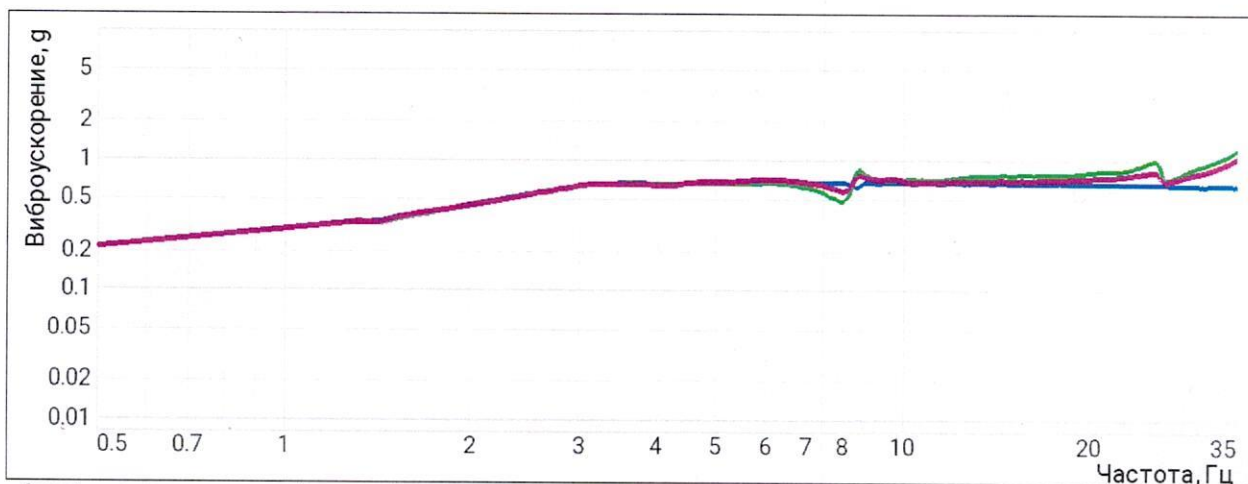
Рисунок А5 – Испытание на сейсмостойкость уровня МРЗ. Направление воздействия, горизонтальное по оси ОУ.
